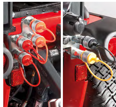
> HYDRAULICKÝ SYSTÉM S JOYSTICKEM
